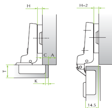
Forgókar 8 féligzárodó pánt
