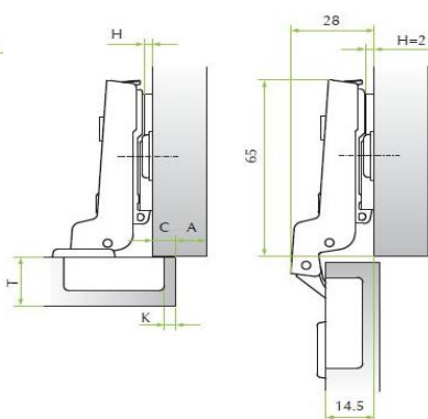
Forgókar 8 félzáró pánt
