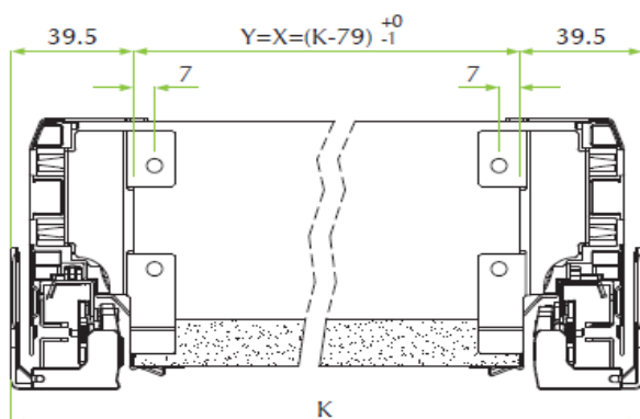
Fa hátsó panel - nézet hátulról
