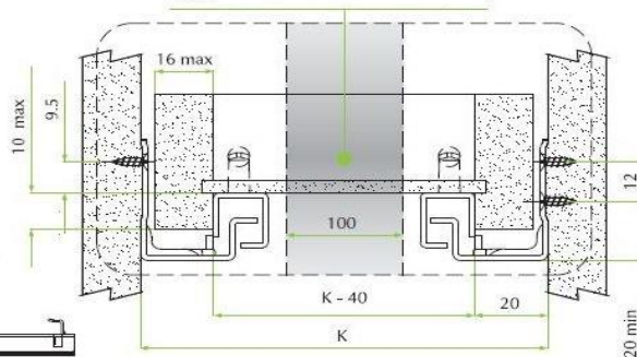
Onetouch aktiválási terület
