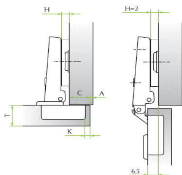
Forgókar 0 rázárodó pánt
