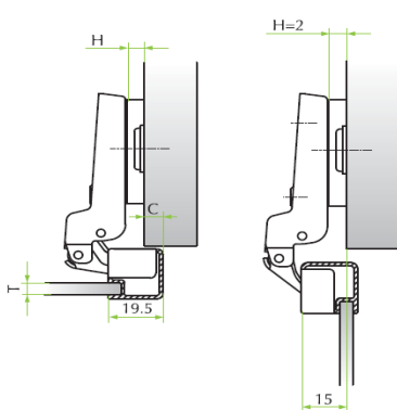
Forgókar 8 féligzáródó pánt
