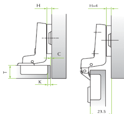
Forgókar 15 közézárodó pánt
