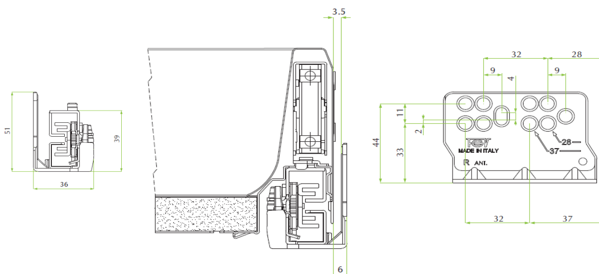
Fióksín méretek és fúrási pozíciók
