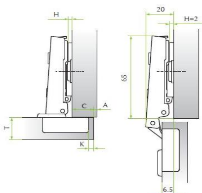
Forgókar 0 rázáró pánt
