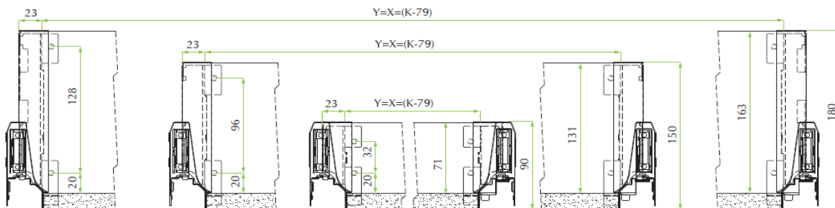
Fa hátsó panel - nézet szemből
