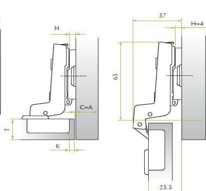
Forgókar 15 közézáró pánt
