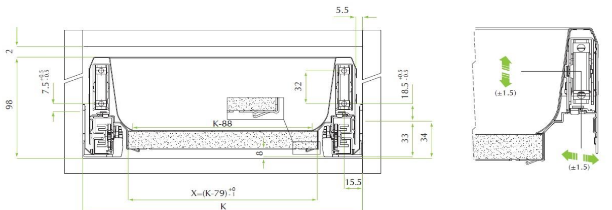
Fióksín méretek és fúrési pozíciók
