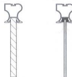
Bútorlap 10 mm Üveg 4 mm + tömítés
