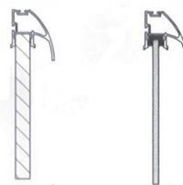
Bútorlap 10 mm Üveg 4 mm + tömítés
